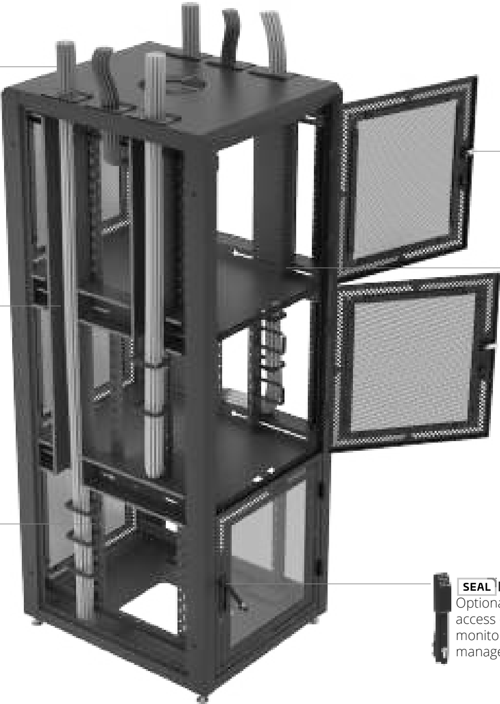
84"H x 30"W x 36"D frame shown
